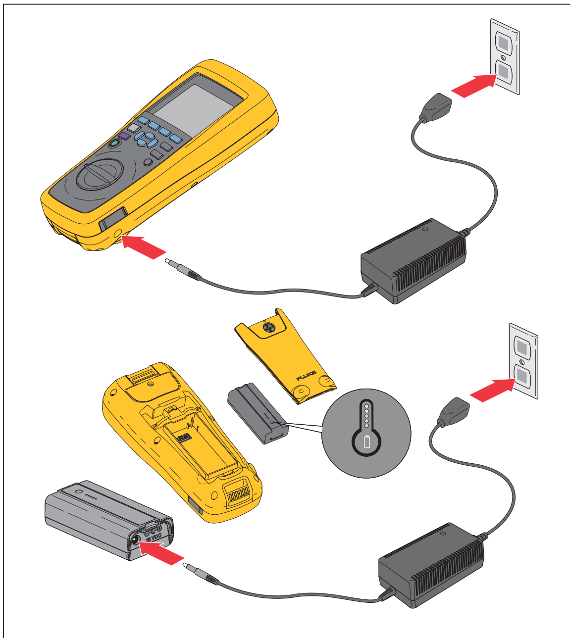
图 6-5. 给电池充电
